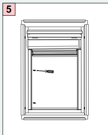
Führungsschienen montage
