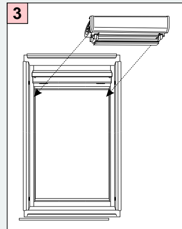
Kassettenmontage
